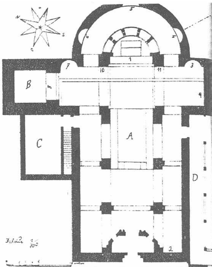
Imatge 5 - Planta de l'església de Sant Pere amb la localització dels altars
